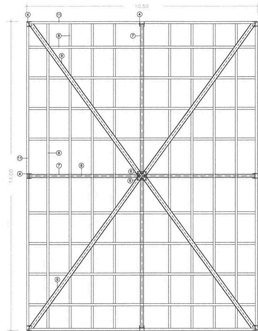
Planta da Estrutura da Cobertura
